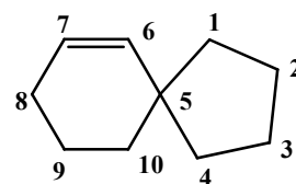
spiro[4,5]dec-6-ène
