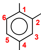
1,2,4-triméthylbenzène
