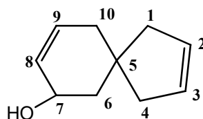
spiro[4,5]dec-2,8-dièn-7-ol
