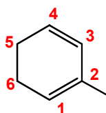
2-méthylcyclohex-1,3diène
