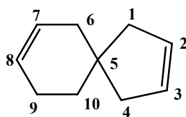
spiro[4,5]dec-2,7-diène
