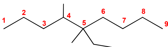
5-éthyl-4,5-diméthyl nonane
