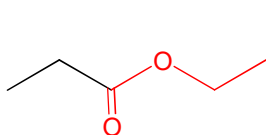
proanoate d'éthyle
