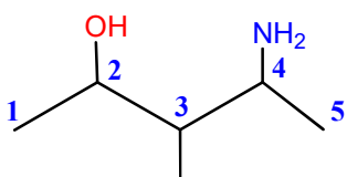
4-amino-3-méthyl pentan-2-ol
