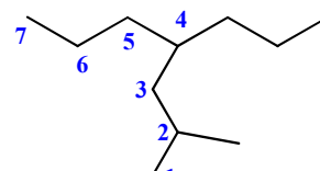
2-méthyl-4-propyl heptane
