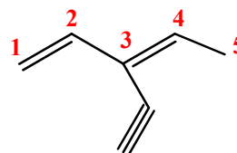
3-éthynyl penta-1,3-diène
