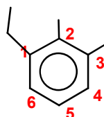
1-éthyl-2,3-diméthylbenzène
