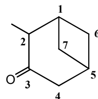
2-méthyl bicyclo[3,1,1]heptan-3-one
