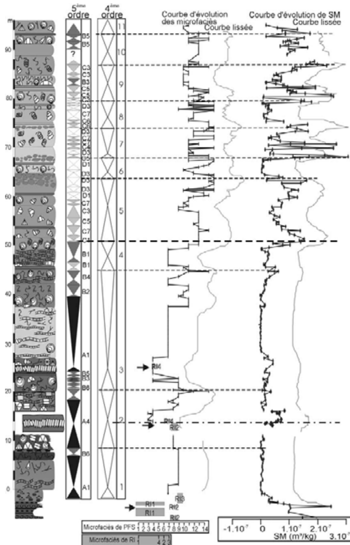
Figure V.7: coupe de référence de Tailfer, cyclicités de quatrième et de cinquième ordre, courbe d'évolution des microfaciès brute et lissée et courbe d'évolution de la SM. Le lien entre l'évolution des microfaciès, la cyclicité et la SM est souligné par les droites pointillées.
