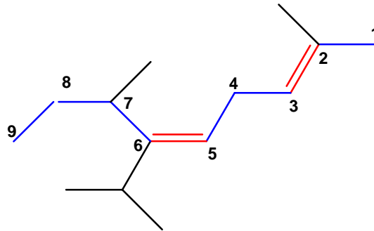
6-isopropyl-2,7-diméthyl nona-2,5-diène
