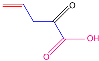
Acide 2-oxopent-4-énoïque
