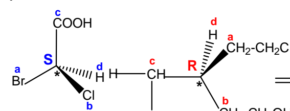
Acide 2-phénylpropanoïque
