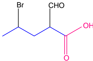
Acide 4-bromo-2-formylpentanoïque
