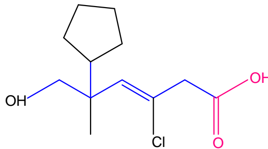
Acide 3-chloro-5-cyclopentyl-6-hydroxy-5-méthylhex-3-énoïque
