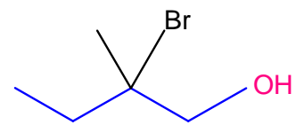
2-bromo-2-méthylbutan-1-ol
