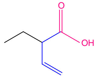
Acide 2-éthylbut-3-énoïque
