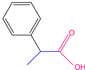
Acide 2-phénylpropanoïque
